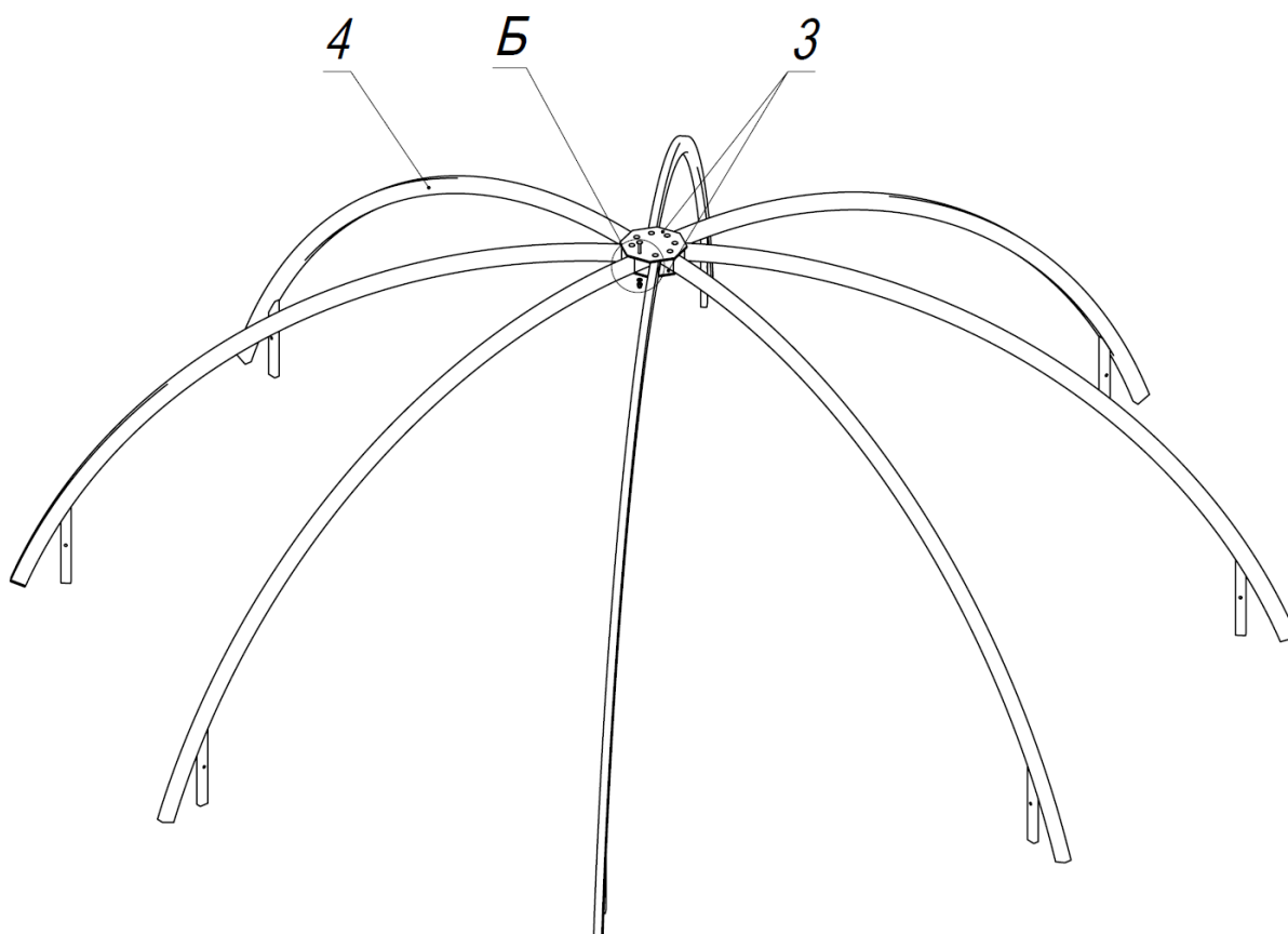
Рис. 2. Сборка крыши.
