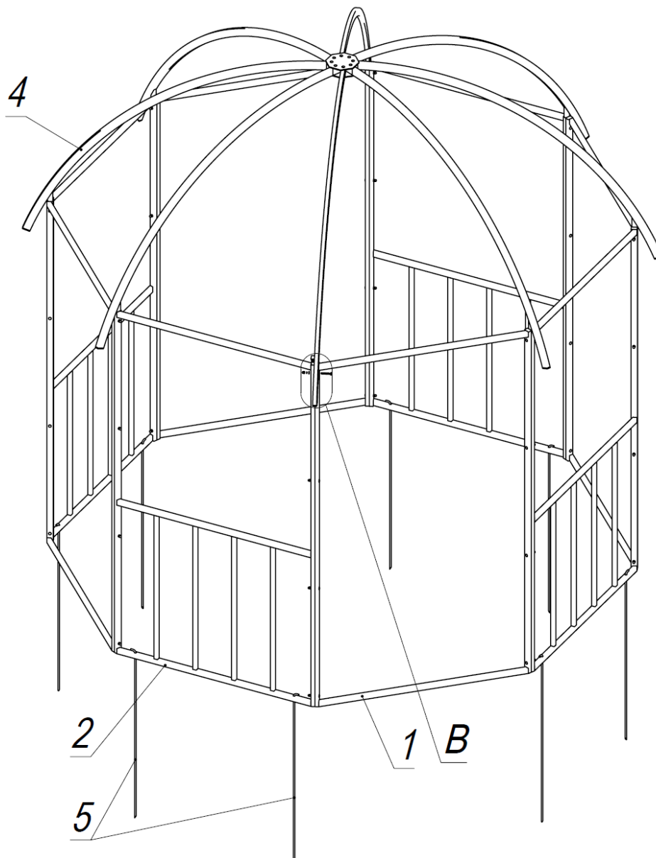
Рис. 3. Установка крыши и кольшков.
